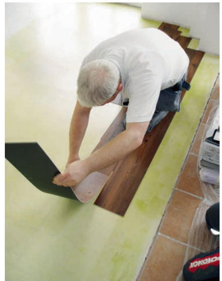
Het leggen van PVC-stroken met behulp van 'iFloor'
